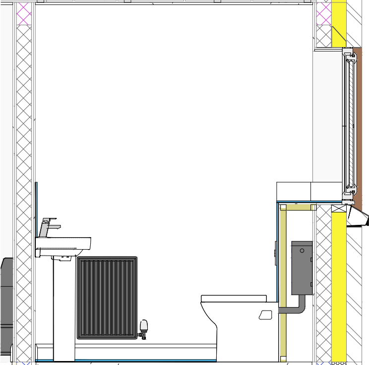
D WC - View D 1 : 25
